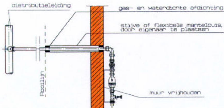
Bovenaanzicht (met bocht)
