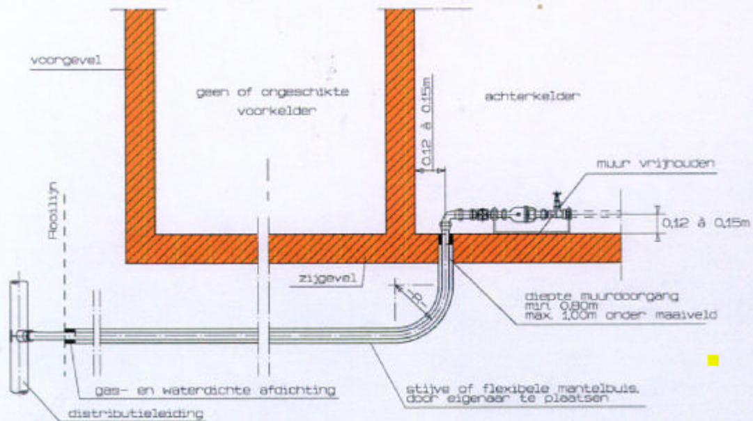
Bovenaanzicht (met bocht)
