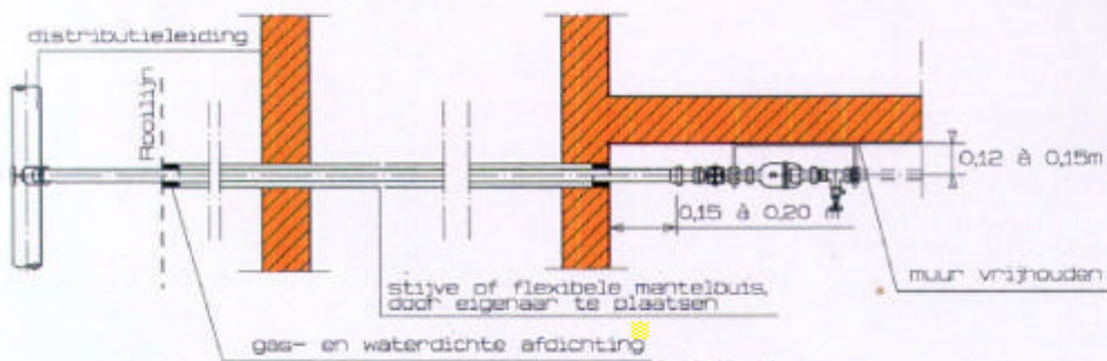
Bovenaanzicht (zonder bocht)
