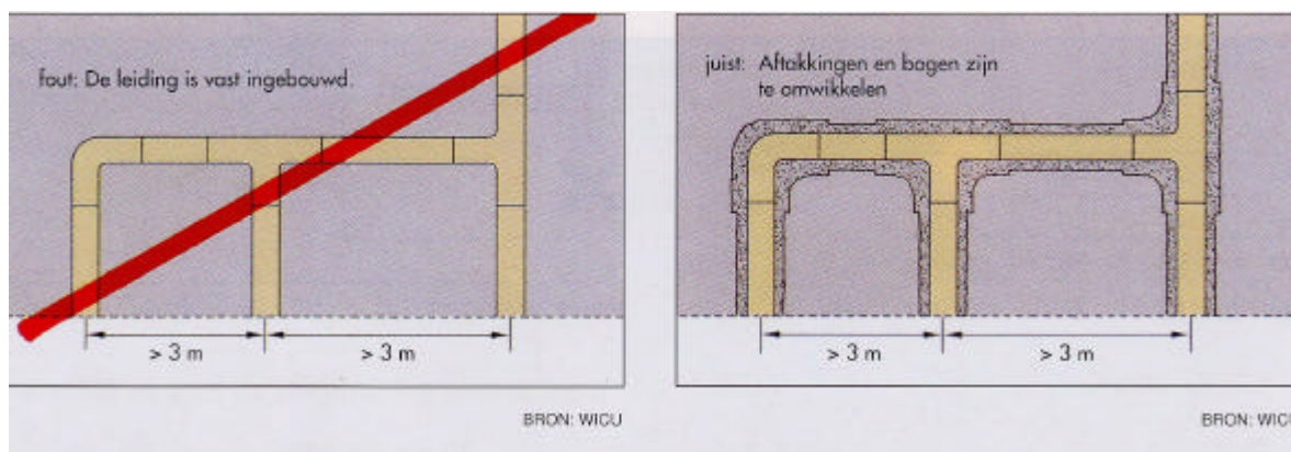
Figuur 3: Foutieve en juiste uitvoering van metalen leidingen in vloeren.
