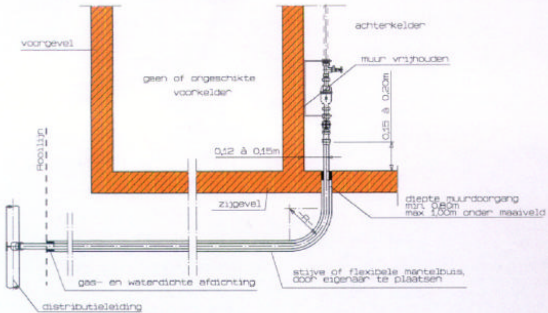
Bovenaanzicht (zonder bocht)
