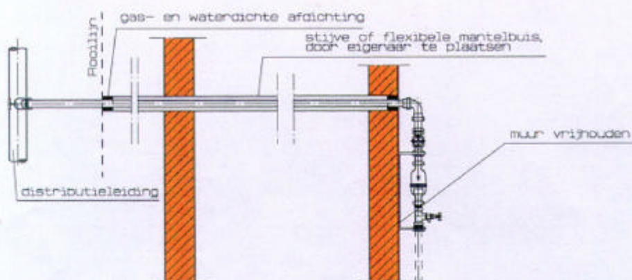
Bovenaanzicht (met bocht)
