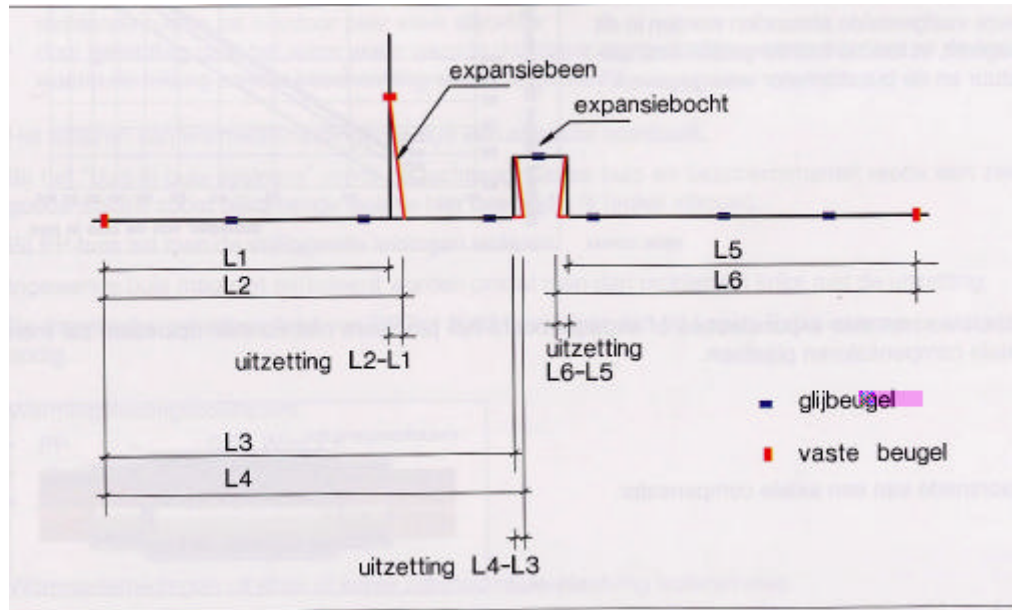
Figuur 4: Voorbeeld van expansiebocht bij vrijliggende leidingen.
